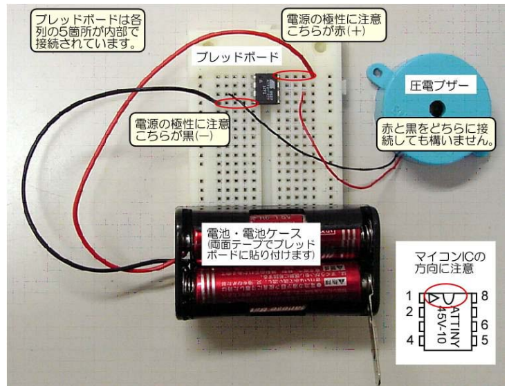
組み立て図
