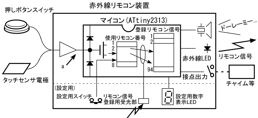
図 2: リモコン装置の構成
